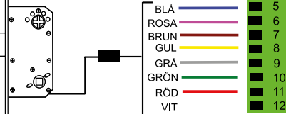
Motorlås 5000 serien
